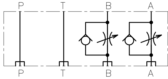
JIS 油圧記号シンボル
